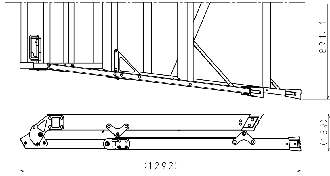
収納状態図
