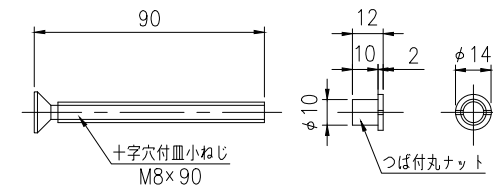
⑥ ボルト・ナット詳細図 S=1/2
