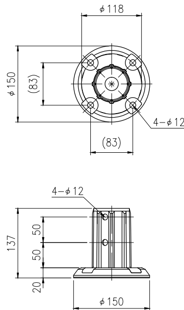
④ ベースプレート詳細図 S=1/5
