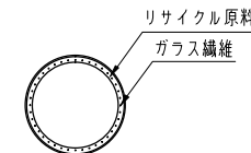
A-A 断面図 S=1/5
