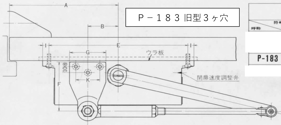
パラレル取付寸法表 (ストップ付)
