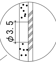
取付孔拡大図
