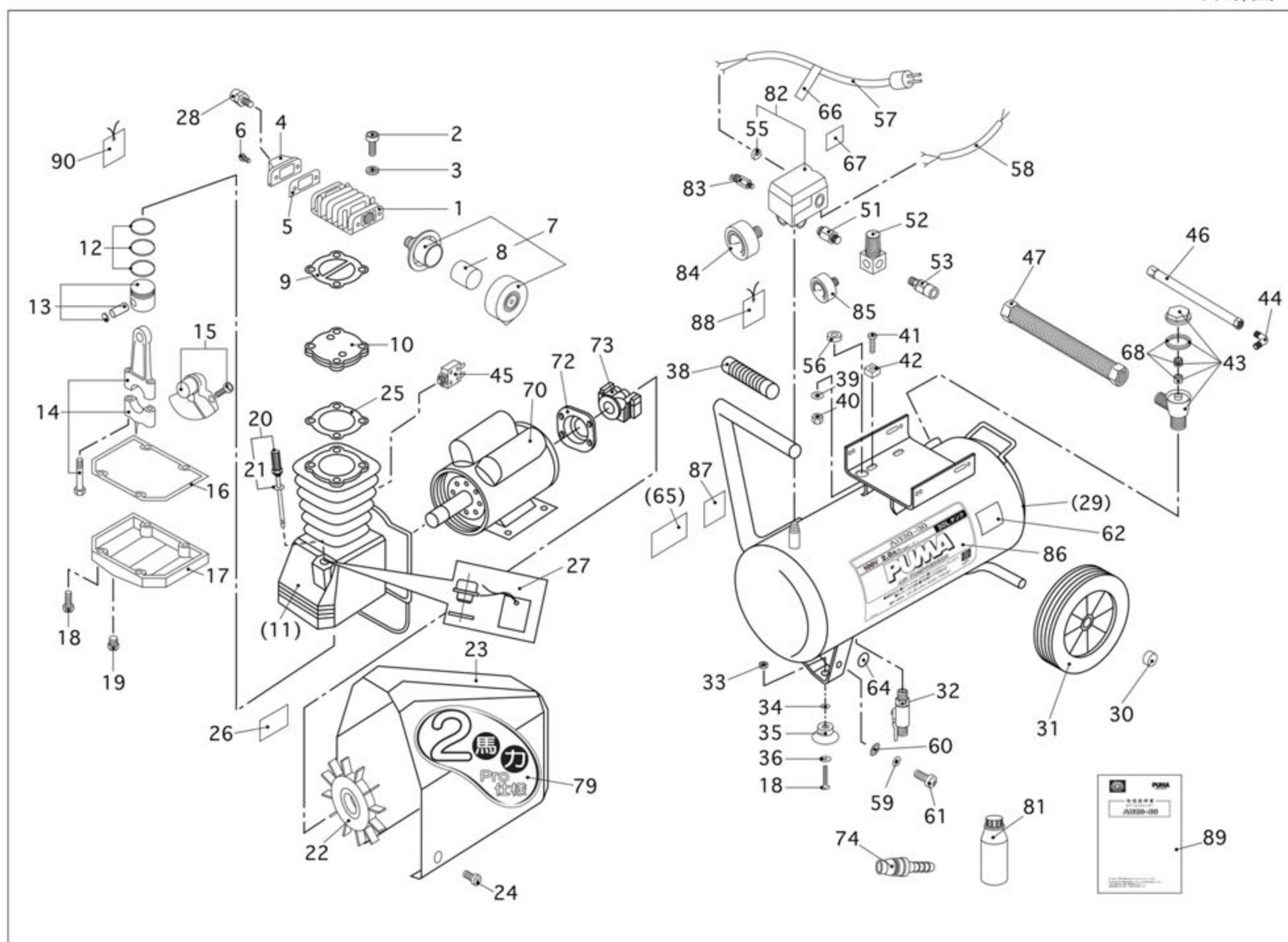
AB20-30 部品表
