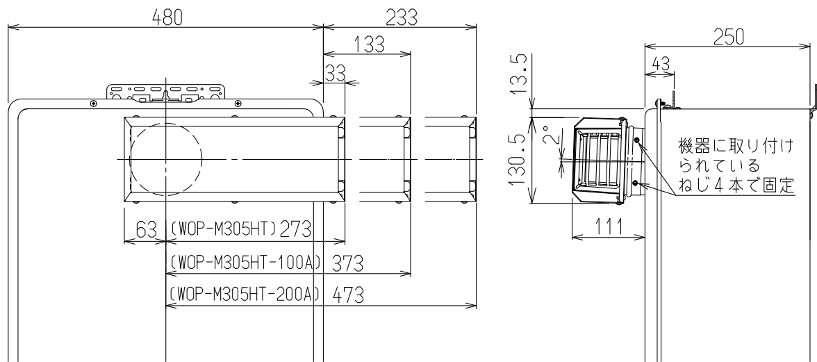
Hタイプに取付けた場合 (尺度フリー)
