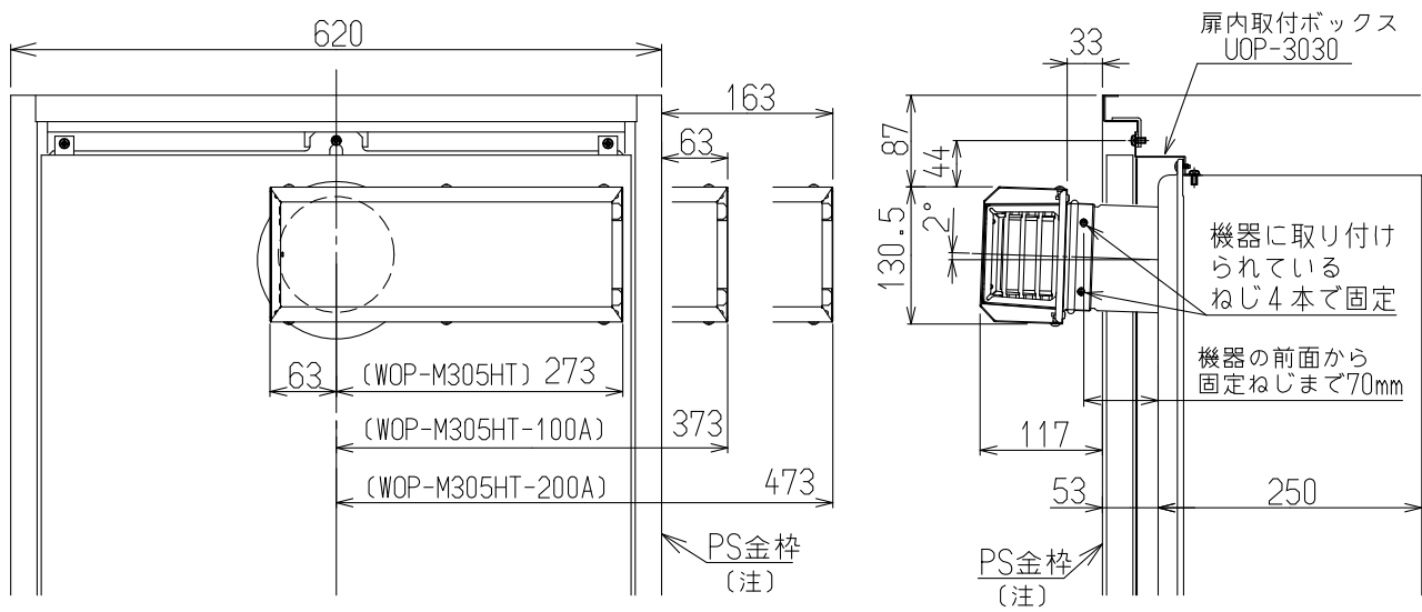
PS(アルコーブ)扉内設置でTタイプに取付けた場合 (尺度フリー)
