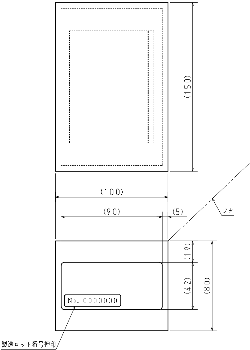
梱包状態図
