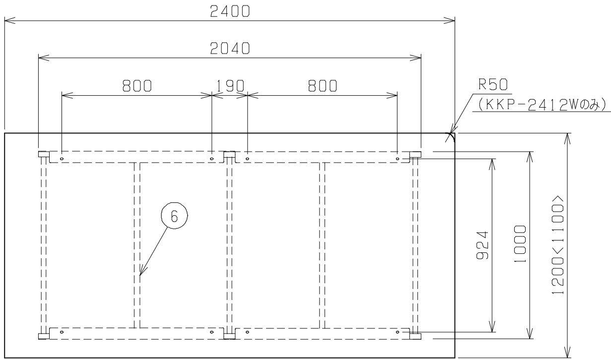
天板・塗装色・中板の有無と品番の関係 W2400×D1200×H740
