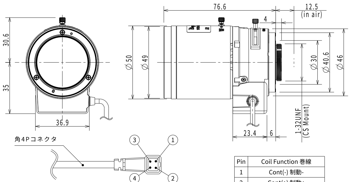
Drawing 外観図面
