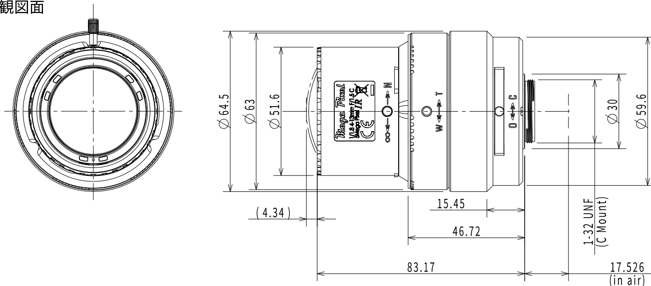
Drawing 外観図面
