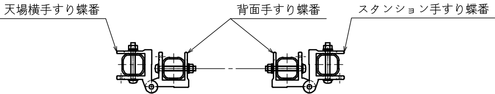
A-A断面 (S=1:5)
