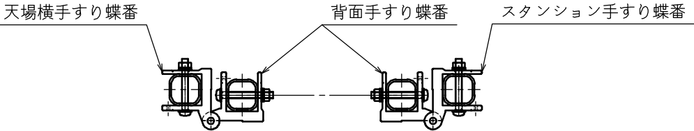
A-A断面 (S=1:5)
