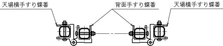
A-A断面 (S=1:5)
