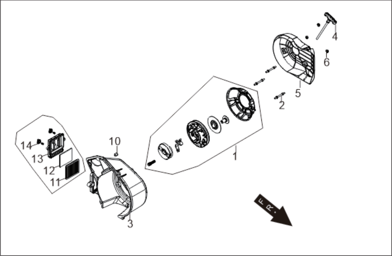
型式名 GV-28IF-AAA-0 (065865401) (5) ファンカバー／リコイルスターター
