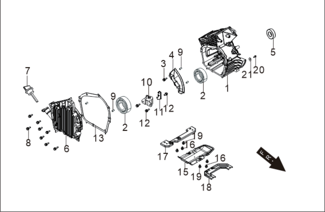
型式名 GV-28IF-AAA-0 (065865401) (1) クランクケース／エンジンベース
