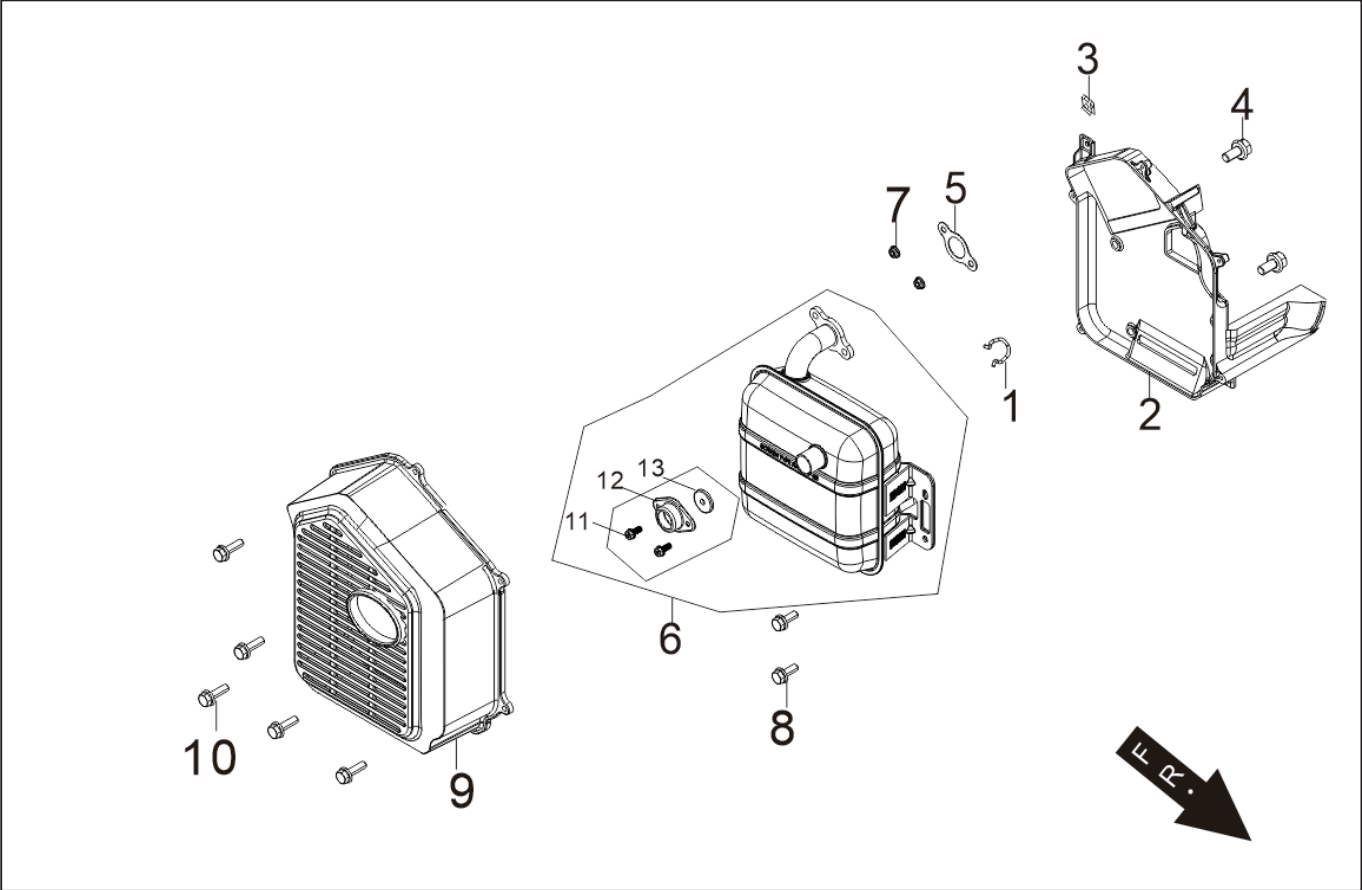
型式名 GV-28IF-AAA-0 (065865401) (8) マフラー
