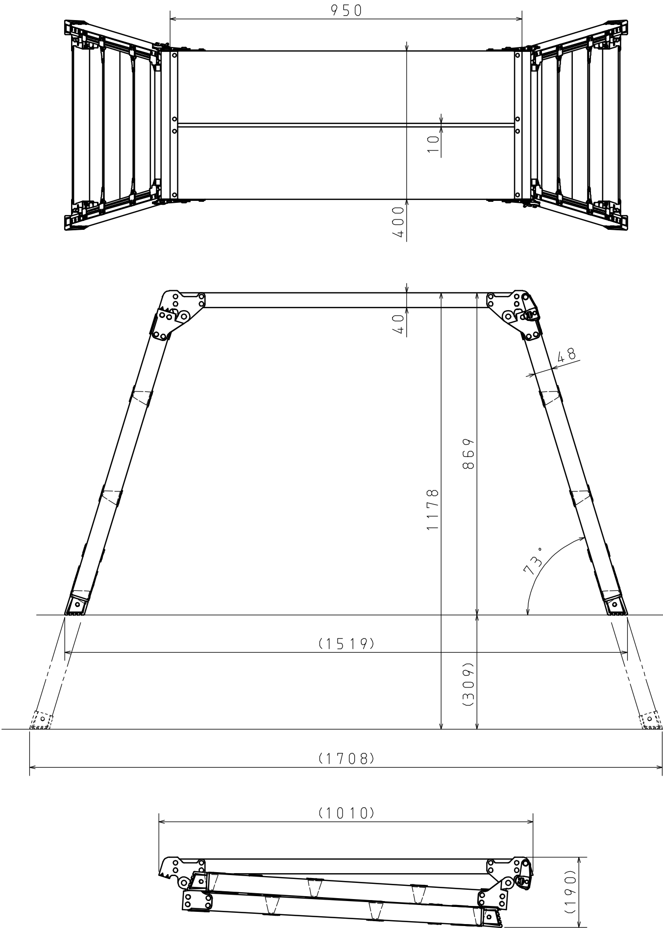
収納状態図
