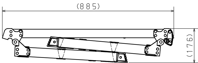
収納状態図
