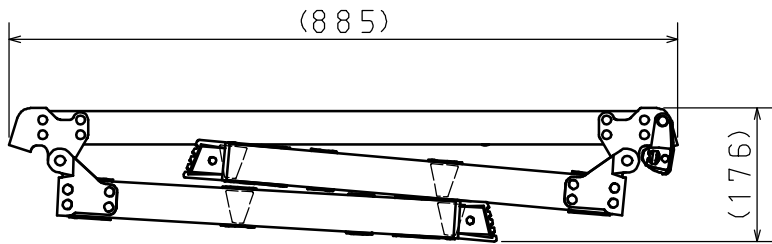
収納状態図
