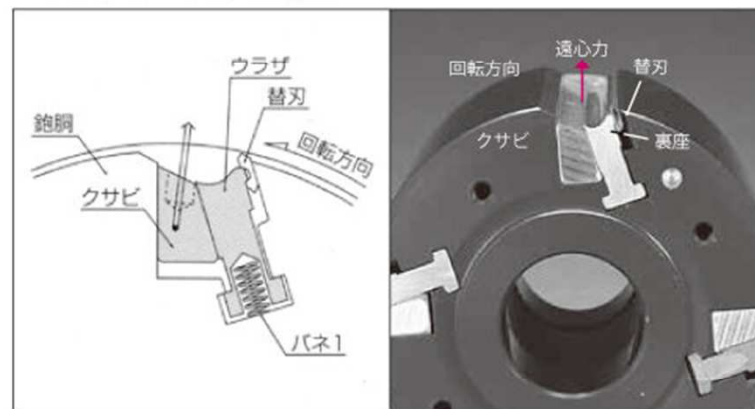
替刃交換の手順(モルダー用)…サイドセット方式
