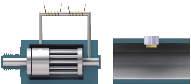
従来のマスフローの構造
