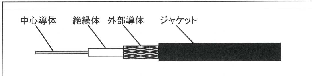
構造図
