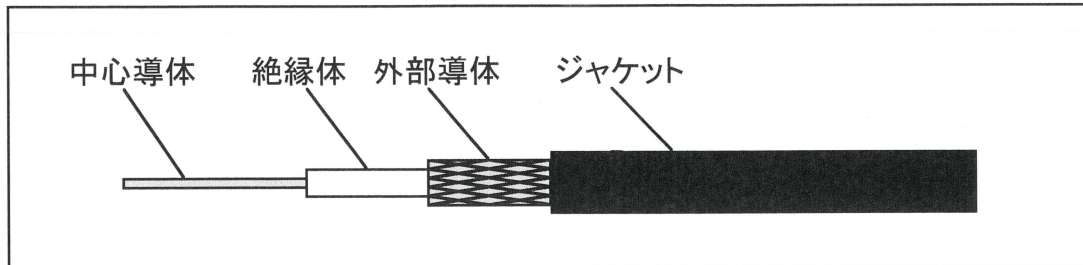
構造図
