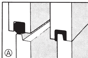
① 凹凸結合方式によるシール
