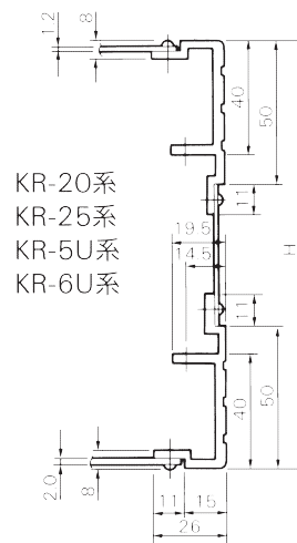
(サイドフレーム断面図)
