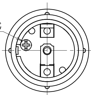
カバー固定ねじ
