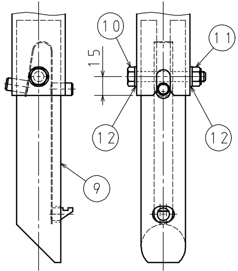
D部詳細 (S = 1 : 3)
