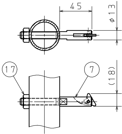
B部詳細 (S = 1 : 3)
