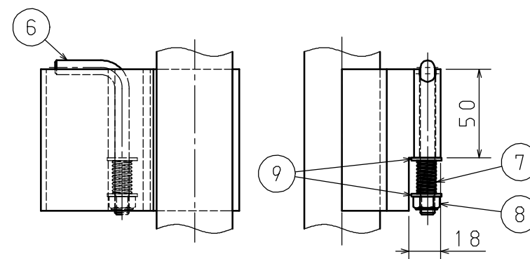
B部詳細 (S = 1 : 3)
