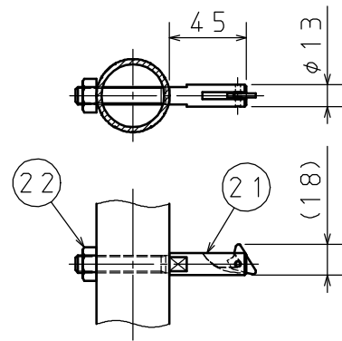
B部詳細 (S = 1 : 4)
