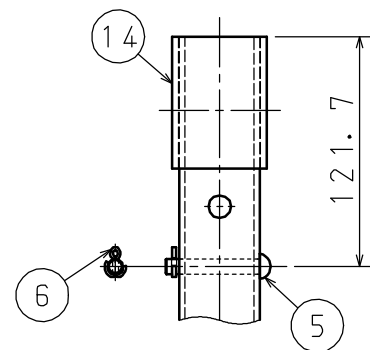
A部詳細 (S = 1 : 4)
