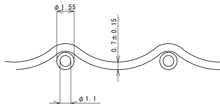
断面詳細
