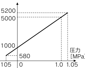
ISE20C-L (正圧用) プロセスデータ
