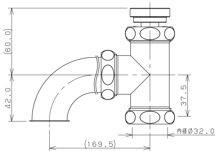
Sトラップの場合
