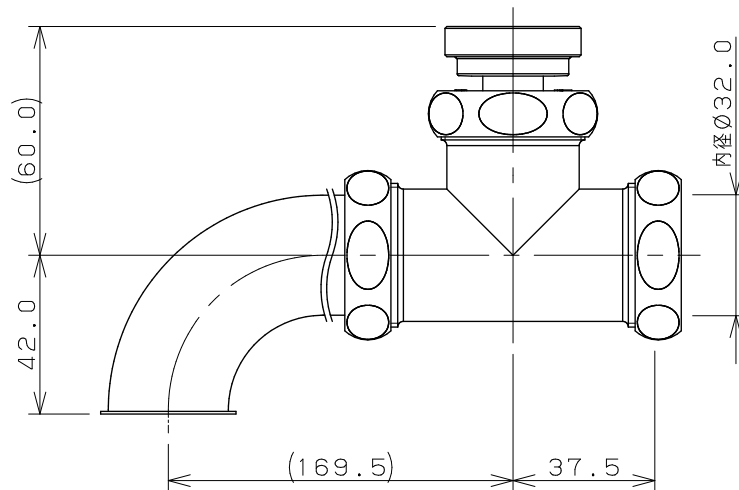
Pトラップの場合
