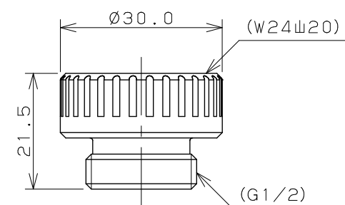
【C】アダプター (TOTO太ホース用)
