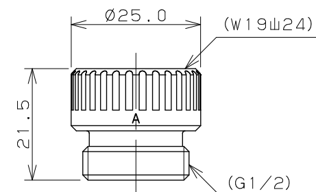
【A】アダプター (TOTO細ホース用)
