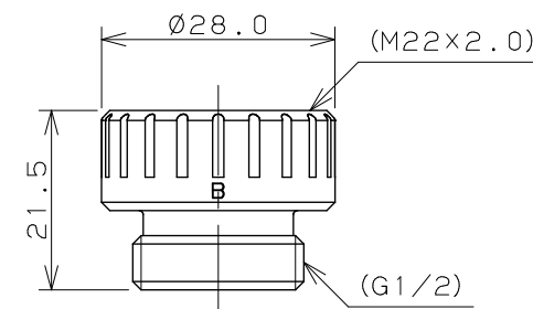
【B】アダプター (KVK用)
