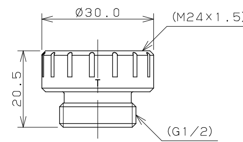
【T】アダプター (TOTO樹脂エルボ用)
