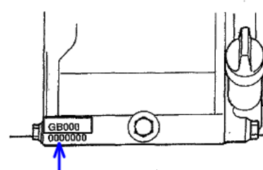
エンジン号機刻印位置
