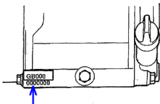
エンジン号機刻印位置
