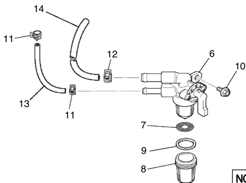
コック
