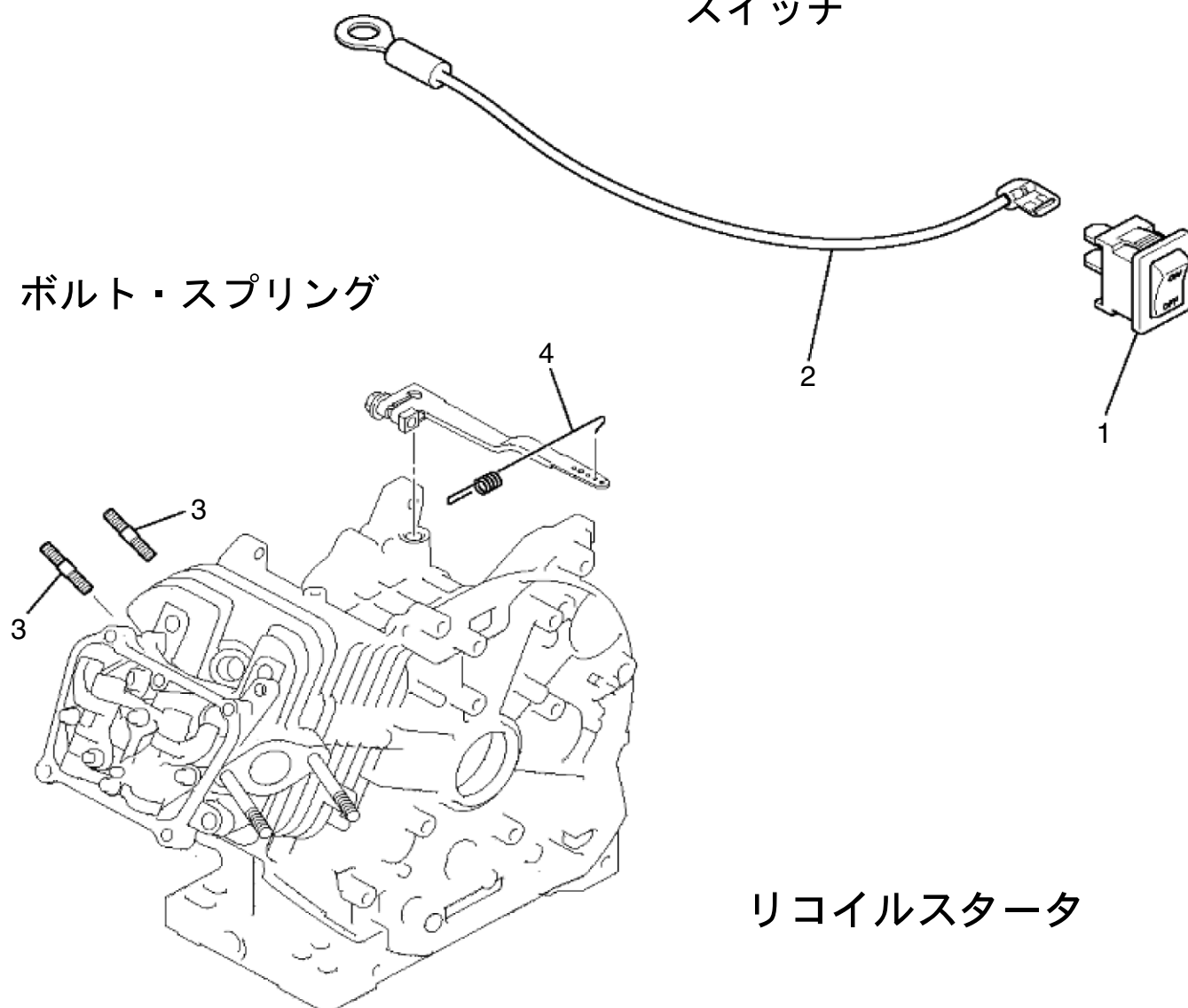
スイッチ
