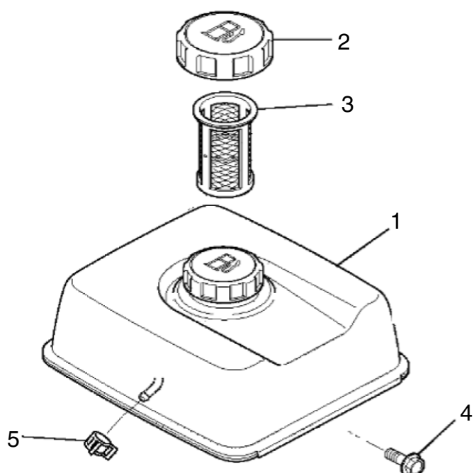
タンク
