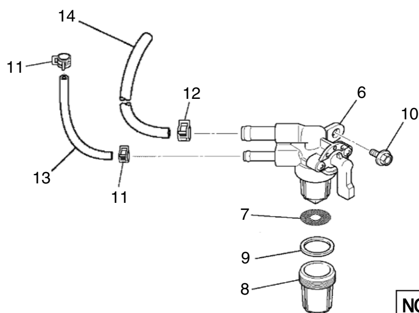
コック
