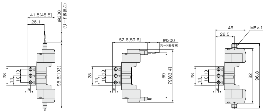
L形プラグコネクタ(L): SYJ3240-□L□□-M5
