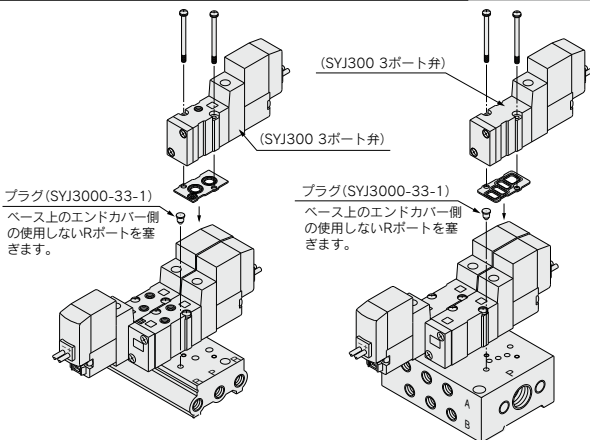
SS5YJ3-20型
