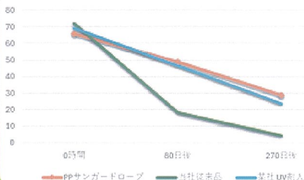
強度低下の推移 (単位kgf)
