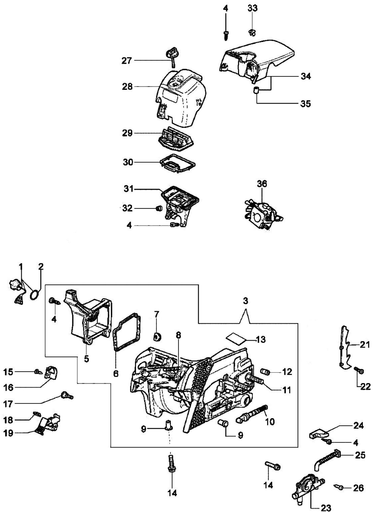
第3図 エンジンケース/エアクリーナー/シリンダーカバー部
