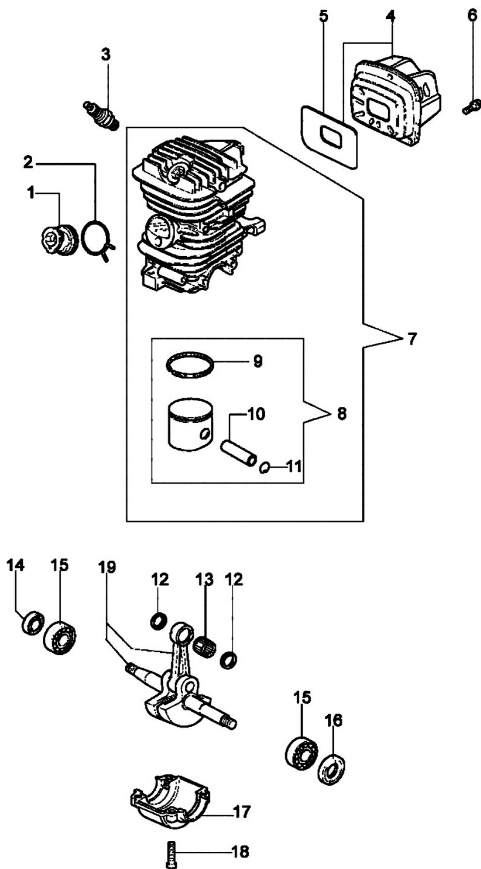
第1図 シリンダー/ピストン/クランクシャフト部
