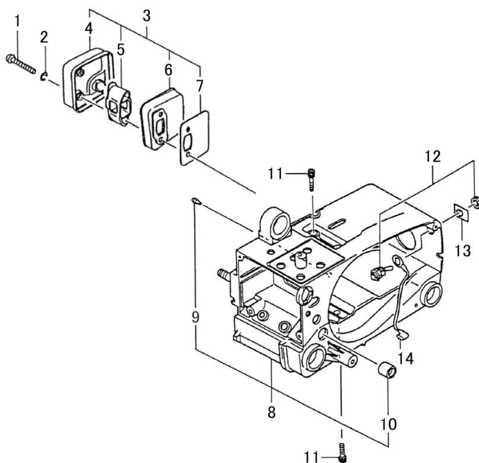
第3図 エンジンケース/マフラー
