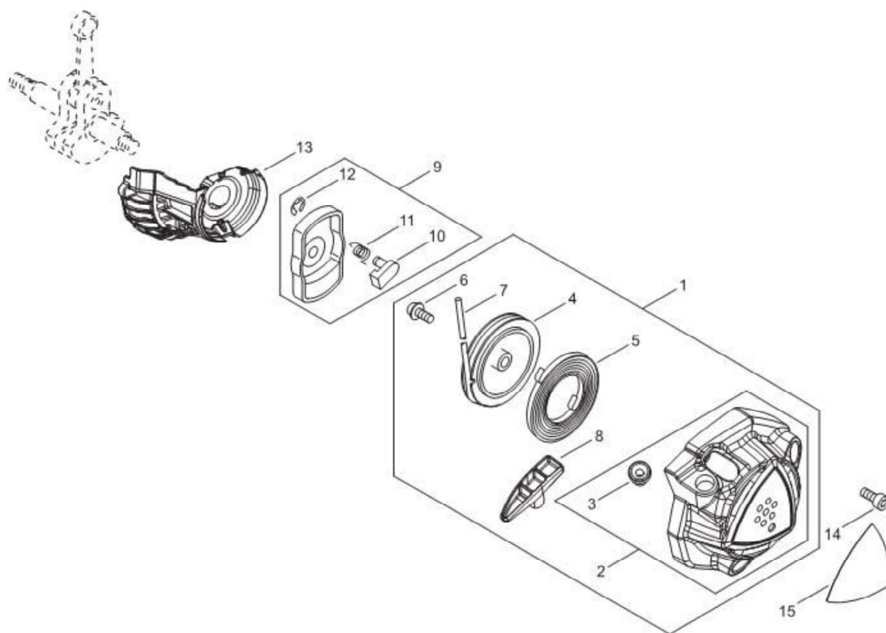
第8図 リコイルスターター・プーリー部
