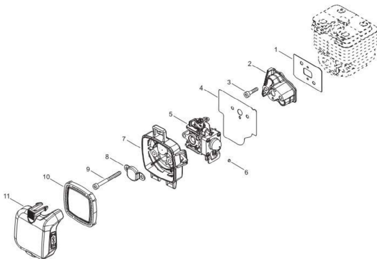
第4図 エアクリーナー・キャブレター部
