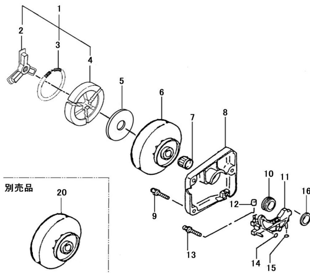
第4図 クラッチ/オイルポンプ
