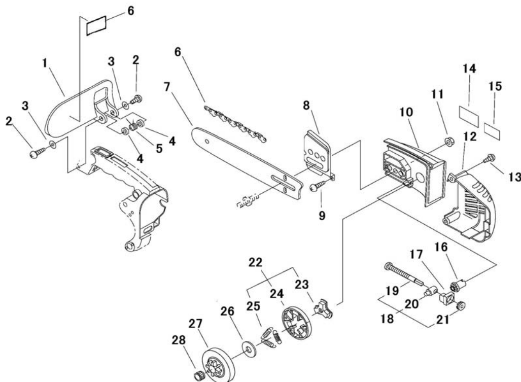
第6図 クラッチ・ガイドバー部
