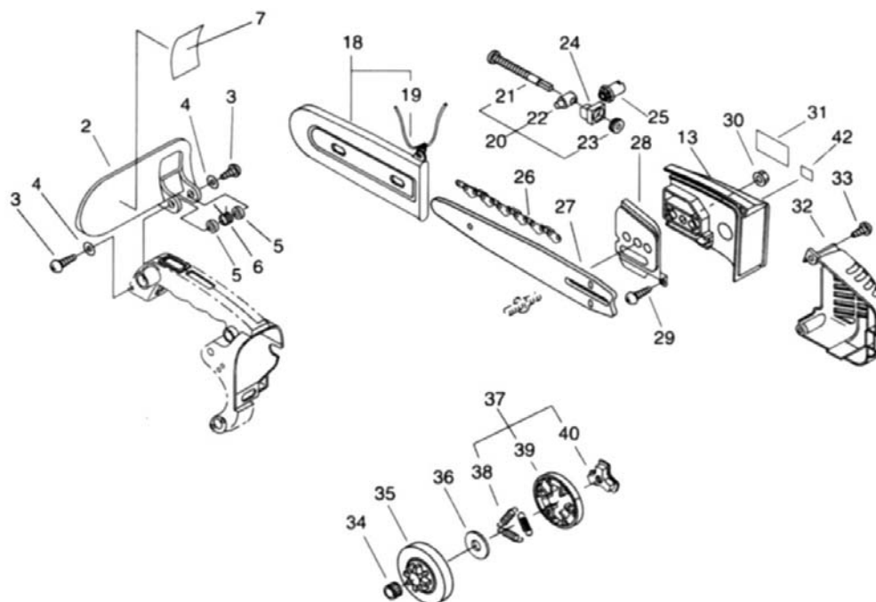
第6図 クラッチ・ガイドバー部
