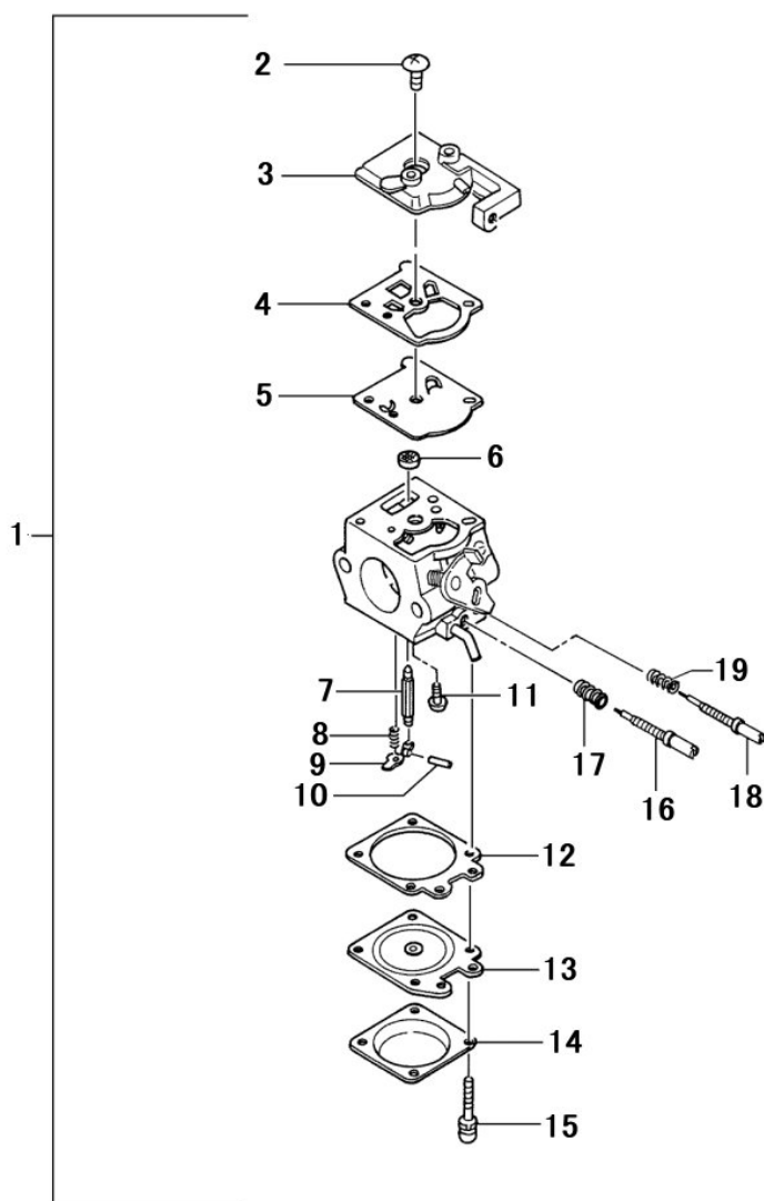
第5図 キャブレター
