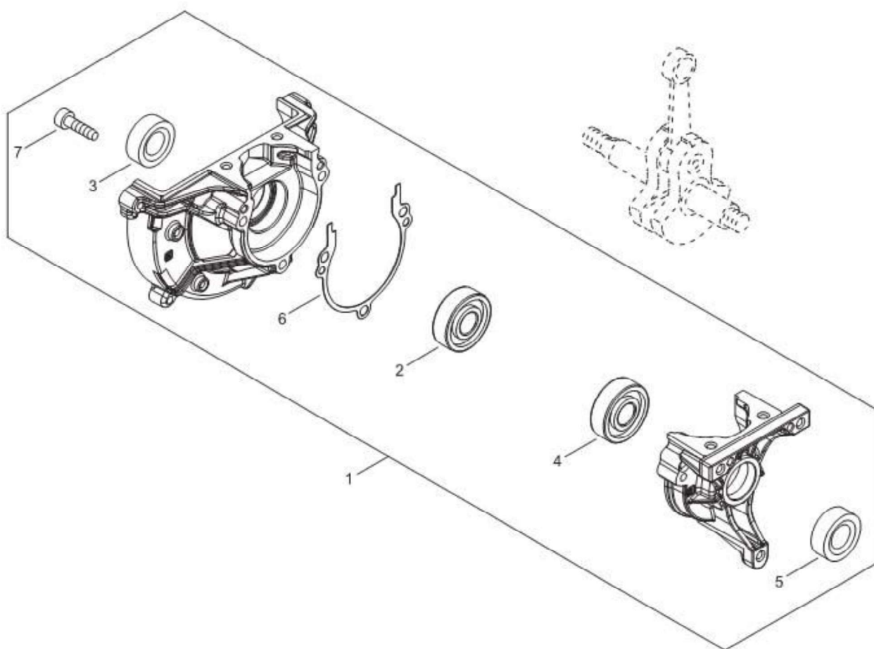
第2図 クランクケース部
