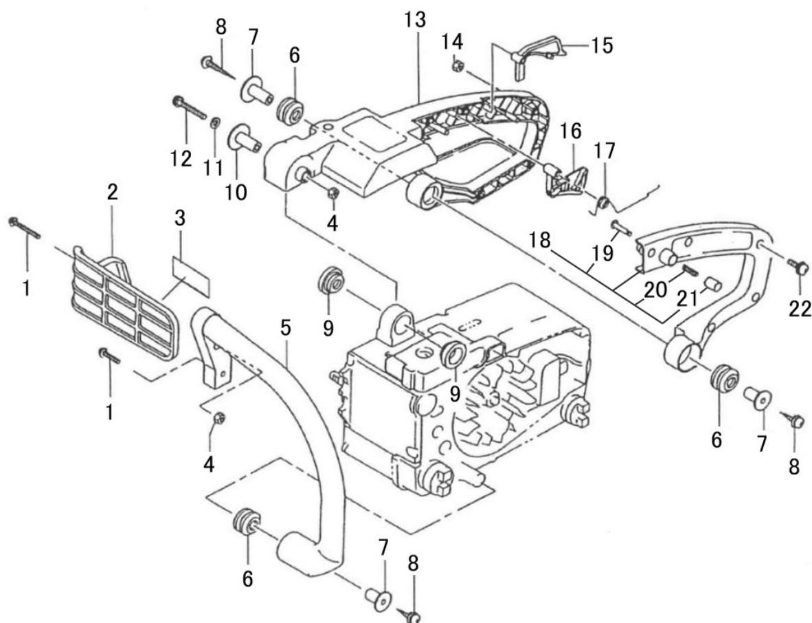
第9図 ハンドル
