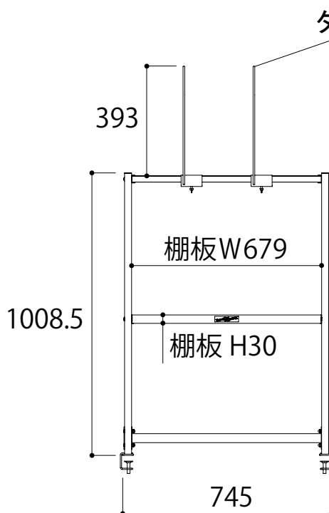
正面図
