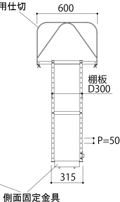
側面図
