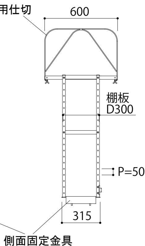
側面図
