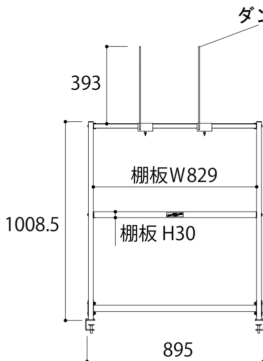
正面図
