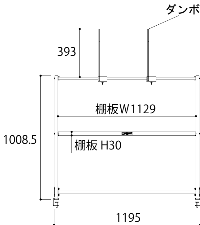
正面図
