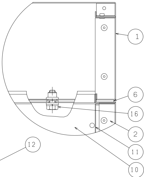
B 部詳細図 (S = 1 / 2 )
