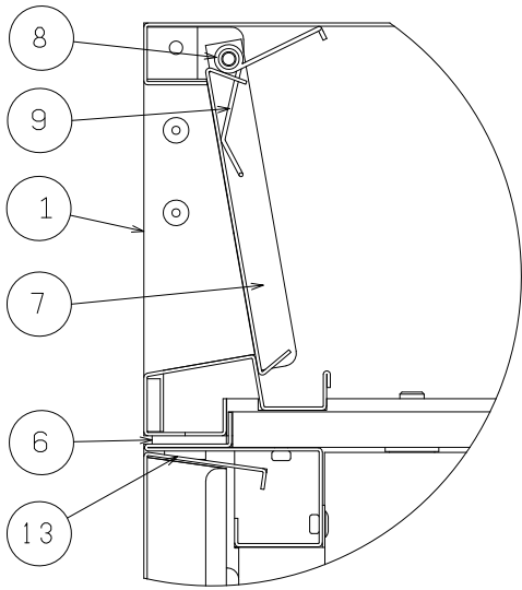
C 部詳細図 (S = 1 / 1 )
