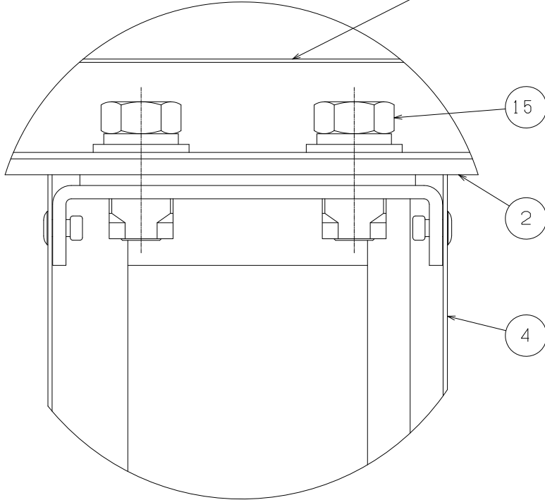
D 部細図 (S = 1 / 1 )
