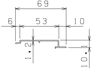
③ 投入口フタ
