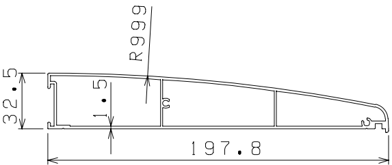
① 正面パネルA
