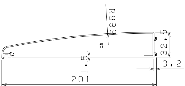
② 正面パネルB
